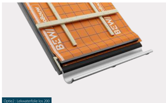
Optie2: Lekwaterfolie los 200
