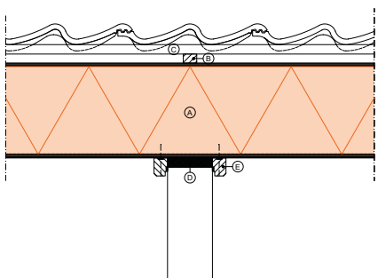
Aansluiting t.p.v. lichte scheidingswand
