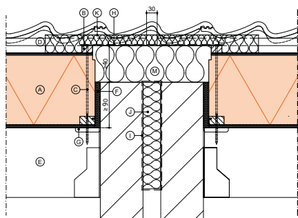
Aansluiting t.p.v. woningscheidende wand
