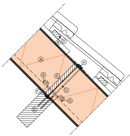
Aansluiting t.p.v. lichte scheidingswand
